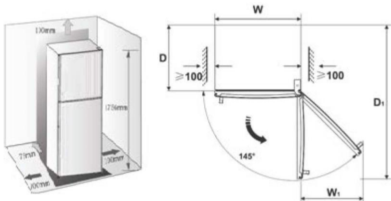
Рисунок-схема рекомендуемого размещения холодильного прибора
