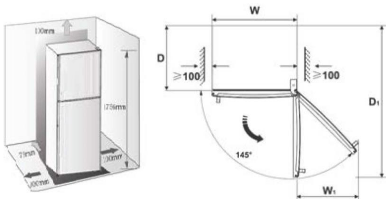
Рисунок-схема рекомендуемого размещения холодильного прибора
